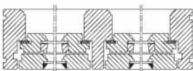
koblede vinduer - vandret snit
