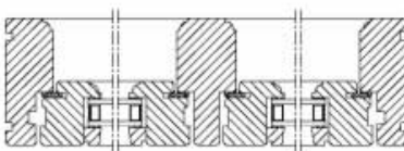
Sidehængt vindue - vandret snit m. post
